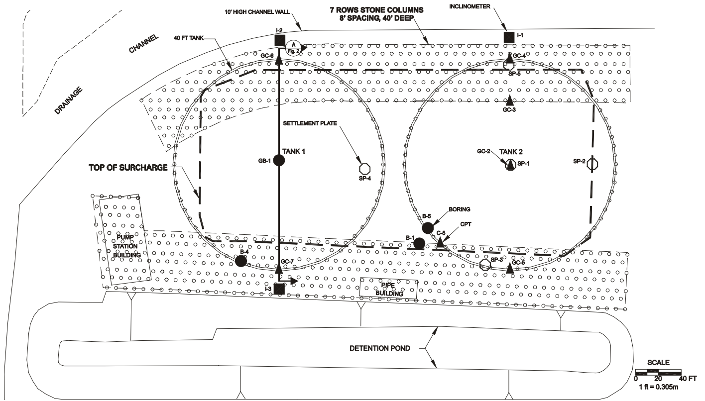
Fig. 1. Site Layout
